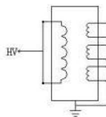
图 7-6 CT 接法
