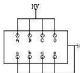
图 7-10 变压器接法
