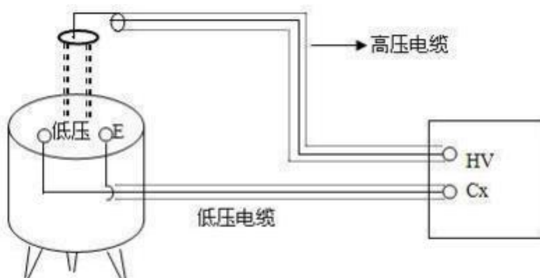
图 7-13 标准电容 BR16 正接线（非接地试品）
