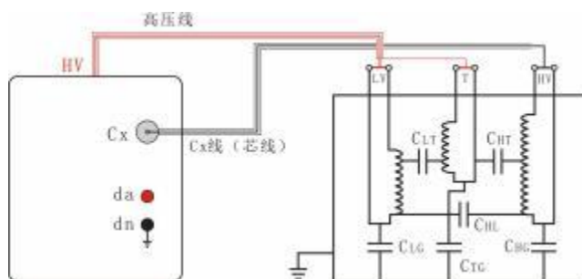
(5)、两绕组变压器 CTG+CHT 测试接线（高压线屏蔽接 LV 绕组）
