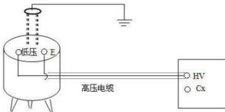
图 7-14 标准电容器 BR16 反接线（接地试品）
