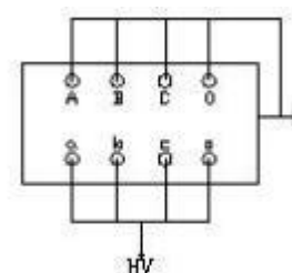
图 7-11 变压器接法
