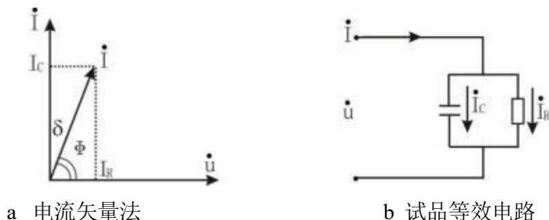
图 5-3 试品等效电路
