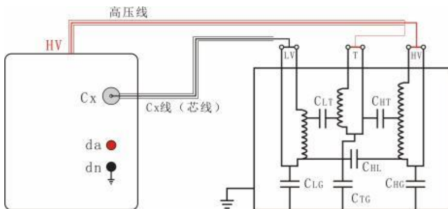
(4)、三绕组变压器 CLG+CLH 测试接线(高压线屏蔽接 HV 绕组)
