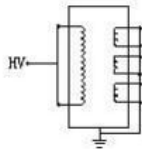
图 7-2 PT 接法
