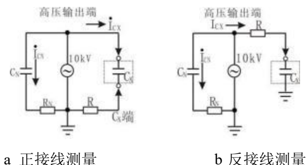
图 5-2 测量原理图
