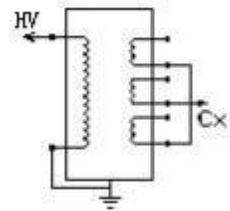
图 7-4 PT 末屏法
